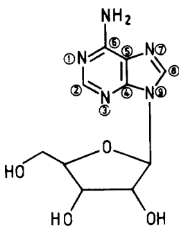
Adenosine
